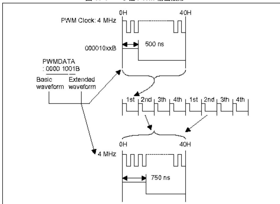
图 11-2 8 位'延伸'波形
