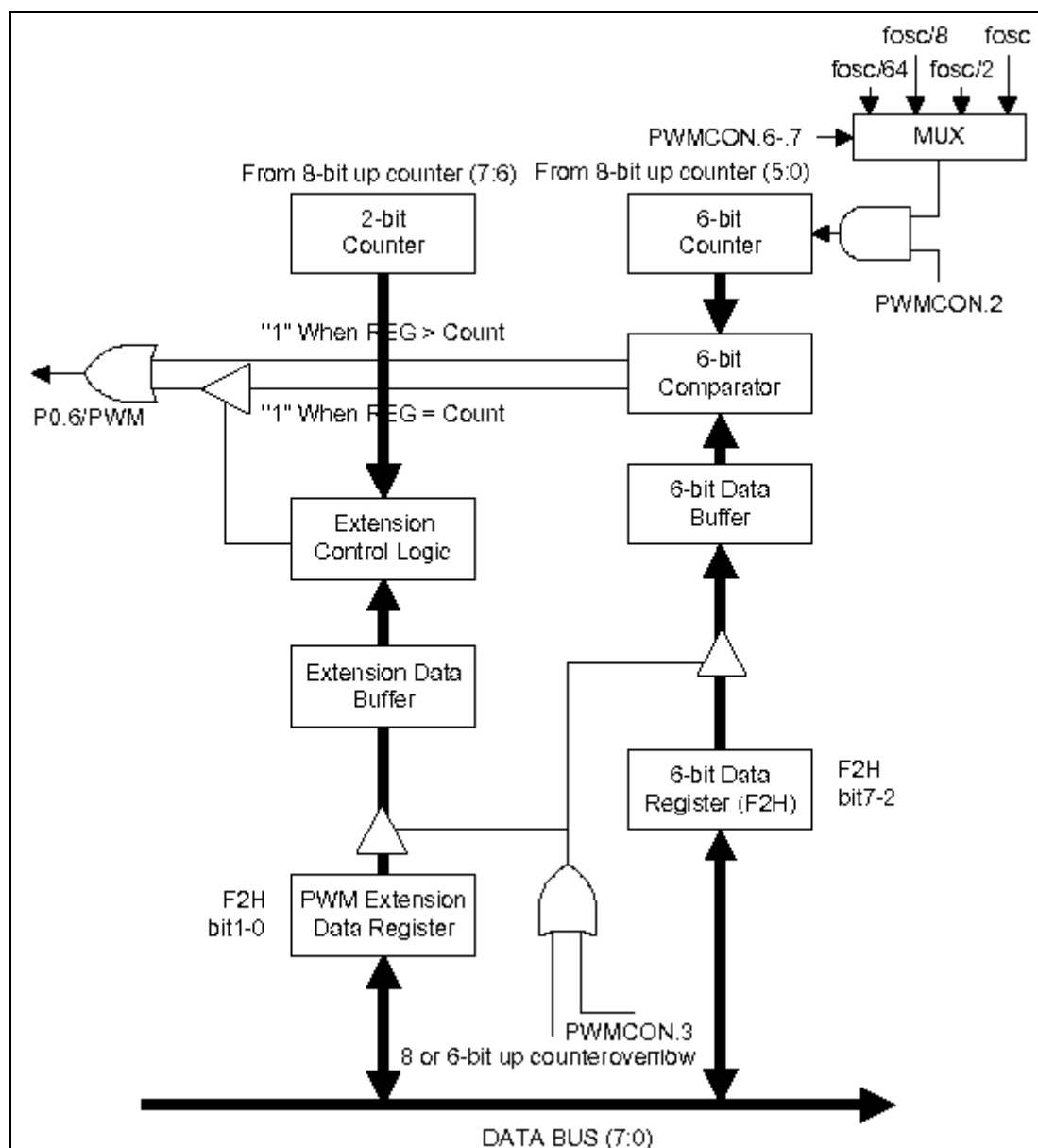
图 11-4 PWM 功能原理图
