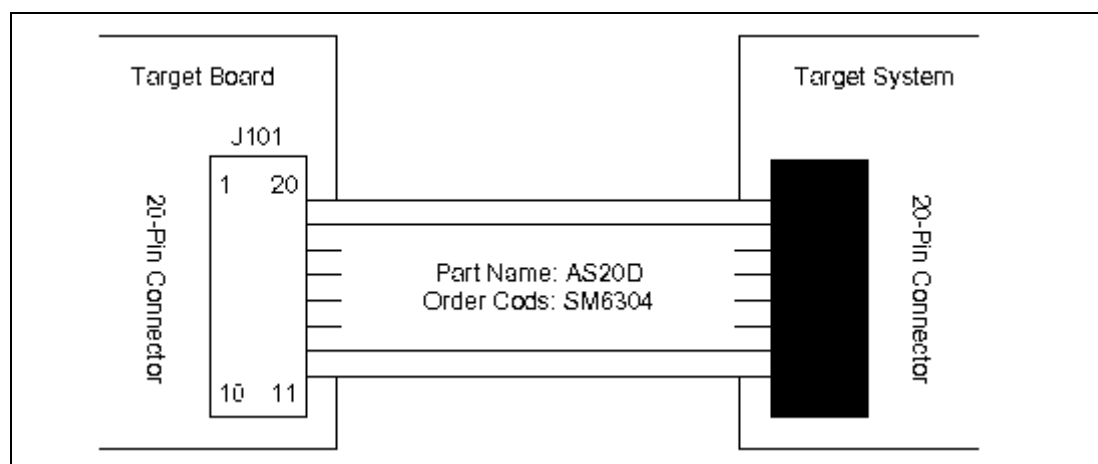
图 16-5 20-DIP 封装 S3C944B/F9454B 适配器
