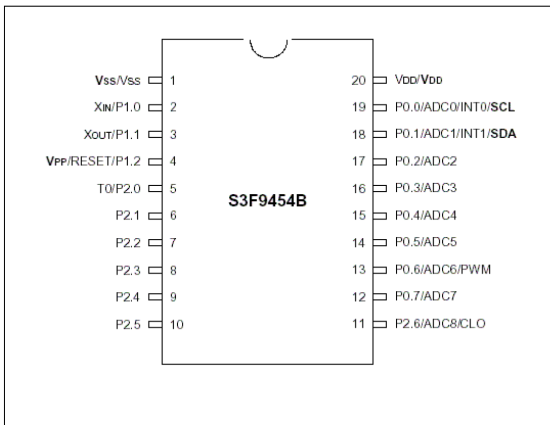
图 15-1 引脚分布图 (20—Pin 封装)
