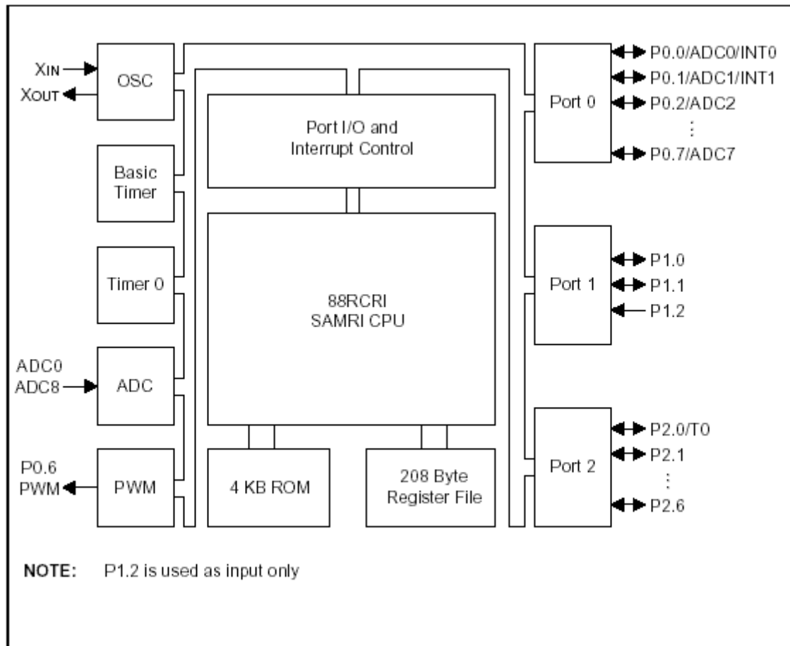
图 1-1 原理图
