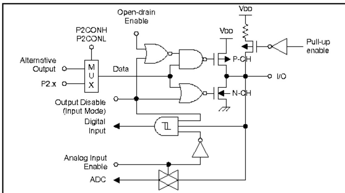
图 1-9 电路类型 E
