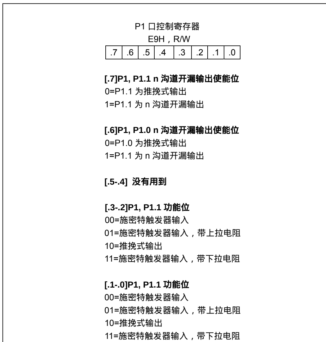
图 9-7 P1 口控制寄存器
