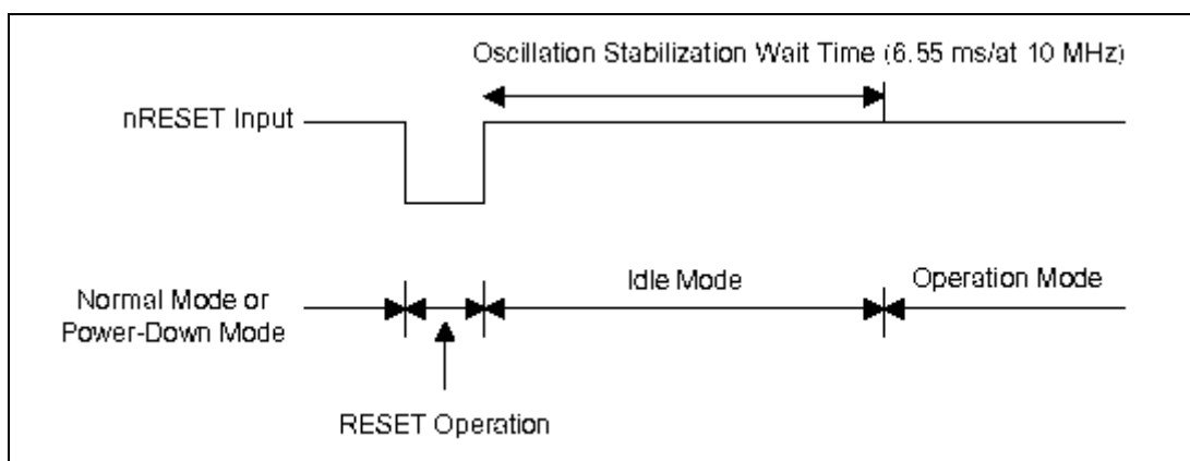
图 8-2 复位后 S3C9454B 的延时原理图
