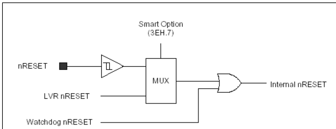
图 8-1 复位电路原理图
