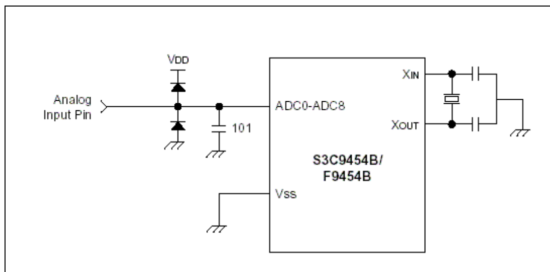
图 12-5 典型 A/D 转换电路
