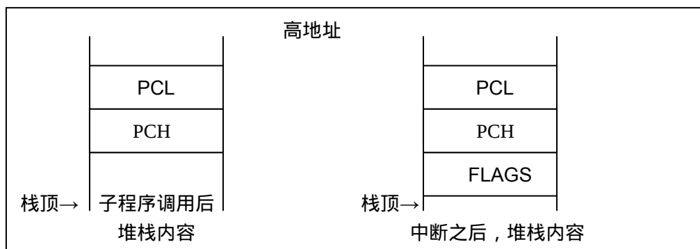
图 2-5 堆栈操作
