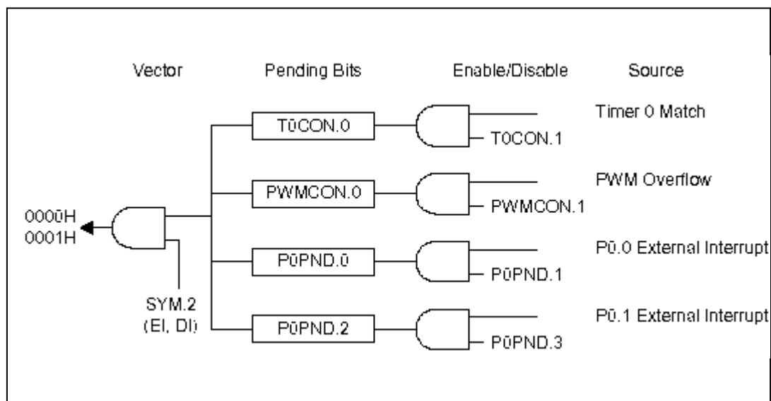
图 5-3 S3C9444/C9454 中断源
