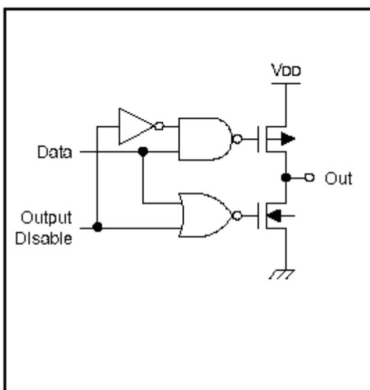
图 1-7 电路类型 C
