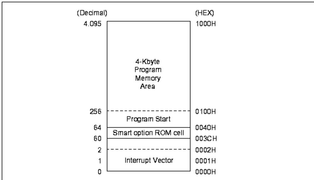
图 2-1 程序地址存贮空间
