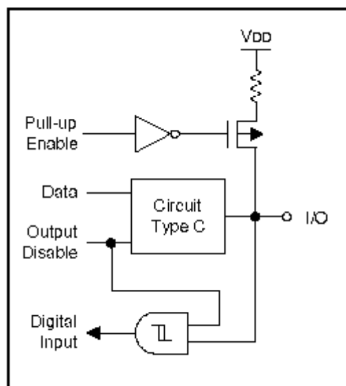
图 1-8 电路类型 D
